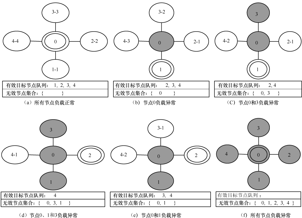
图 5 典型工作场景机制和原理
