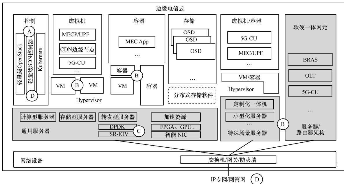
图 1 边缘电信云内部架构
